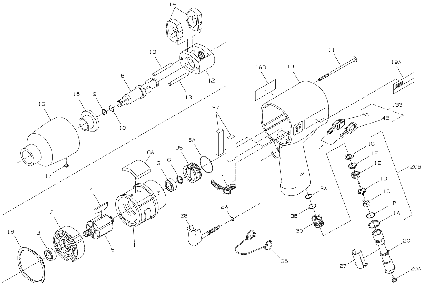
(Dwg. TPA1476-1)
