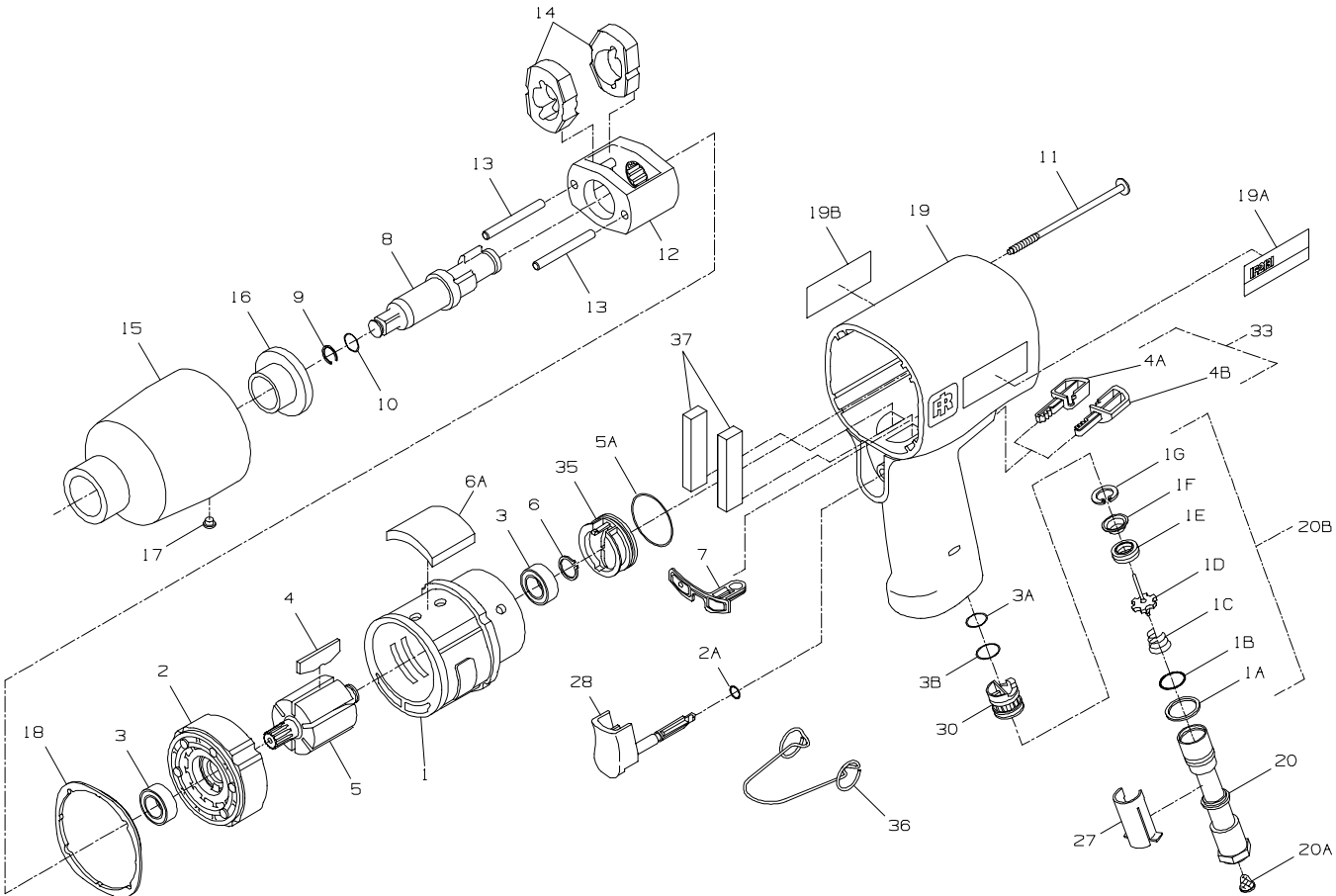
(Dwg. TPA1476-1)
